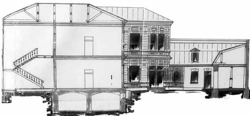
Слева и сверху: проект деревянного 2-х этажного дома на Самарской улице (автор Ф. П. Засухин). Внизу: городская усадьба Тимротов (Самарская, 165), фото 2002 года.
